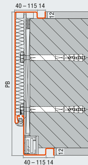
2-schalige Umfassungszarge Individuell Dübelmontage ab 250 mm Profilbreite Beton / Mauerwerk mit Option Schattennut
