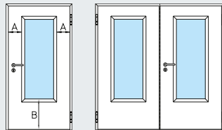
Verglasung Bild 3
