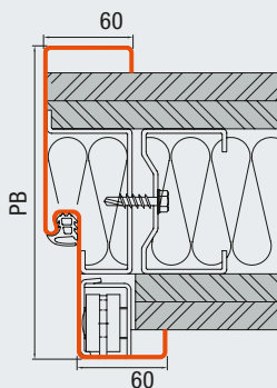
Umfassungszarge 60 für wandbegleitenden Einbau (Abb. Metallständerwerk)
