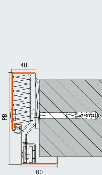
Umfassungszarge 60 Standard Dübelmontage bis 250 mm Profilbreite Beton / Mauerwerk (Standard)
