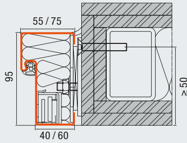
Blockzarge 95 / 55, 95 / 75 Schraubmontage, flächenbündige Wandmontage, Bandseite (Abb. Metallständerwerk)
