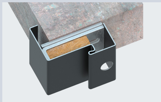
1. Zarge in die Öffnung stellen und ausrichten
