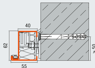
Blockzarge 62 / 55 Dübelmontage, flächenbündige Wandmontage, Bandgegenseite Beton / Mauerwerk
