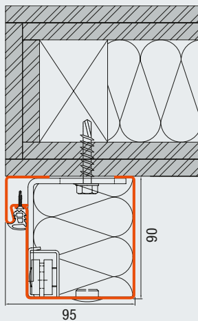
Rahmenzarge (nur MZ-Türen) Schraubmontage (Abb. Holzständerwerk)
