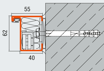
Blockzarge 62 / 55 Dübelmontage Beton / Mauerwerk (Standard)
