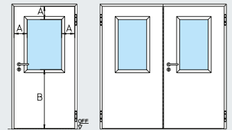
Verglasung Bild 2
