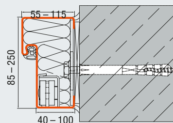
Blockzarge Individuell Dübelmontage Beton / Mauerwerk
