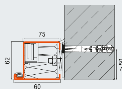
Blockzarge 62 / 75 Dübelmontage, flächenbündige Wandmontage, Bandgegenseite Beton / Mauerwerk
