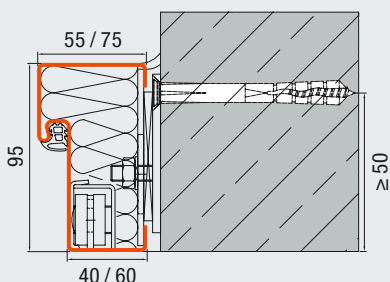
Blockzarge 95 / 55, 95 / 75 Dübelmontage, flächenbündige Wandmontage, Bandseite Beton / Mauerwerk
