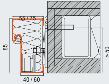
Blockzarge 85 / 55, 85 / 75 Schraubmontage, flächenbündige Wandmontage, Bandseite (Abb. Metallständerwerk)
