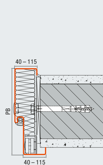
Umfassungszarge Individuell Beton / Mauerwerk
